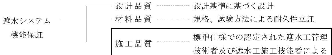
図1. 遮水システム機能保証概念図
